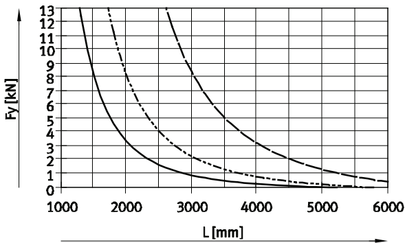
Сила Fy
