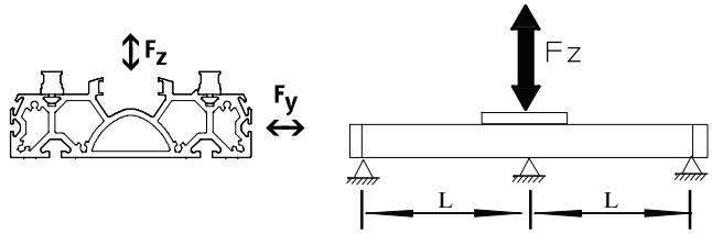
Сила Fz
