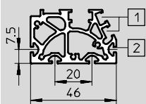
Размер 50
